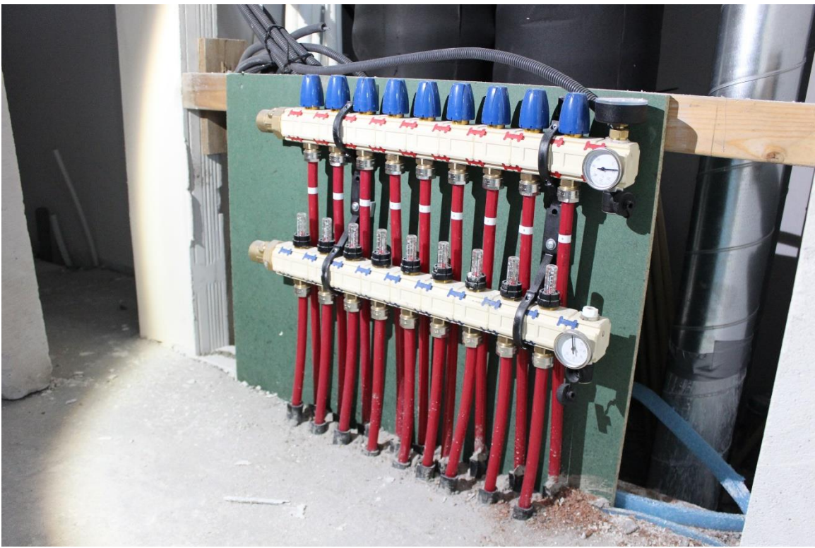
Vloerverwarming
